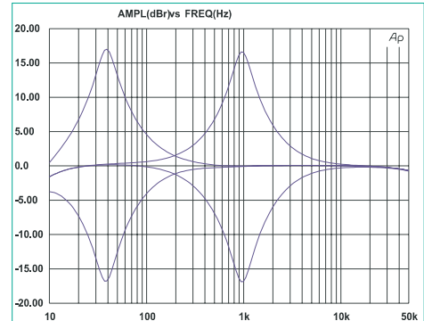
СЧ эквалайзер MF2
