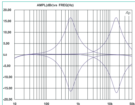
СЧ эквалайзер MF1
