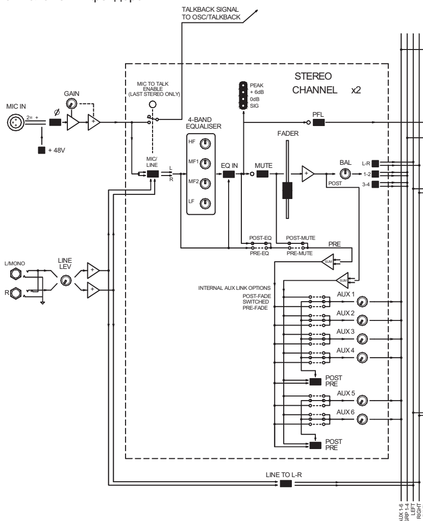
Схема стереоканала показывает маршрутизацию сигналов двусторонней связи и линейного стереосигнала.
