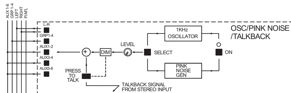
Схема секции генератора и двусторонней связи.
