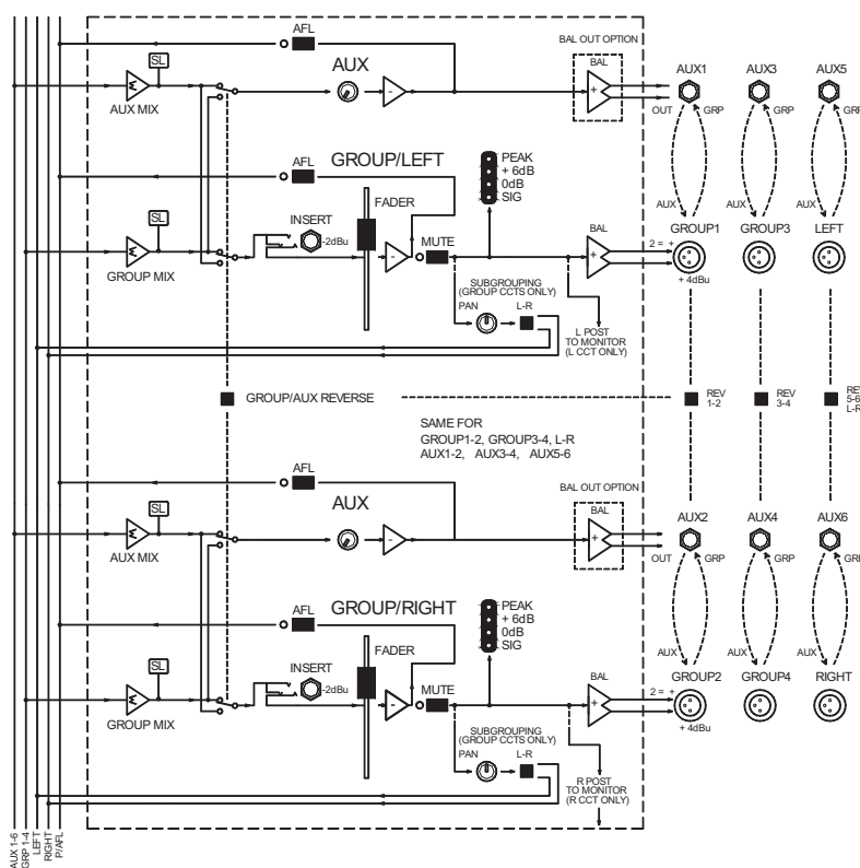
Схема маршрутизации сигналов групп и посылов.
