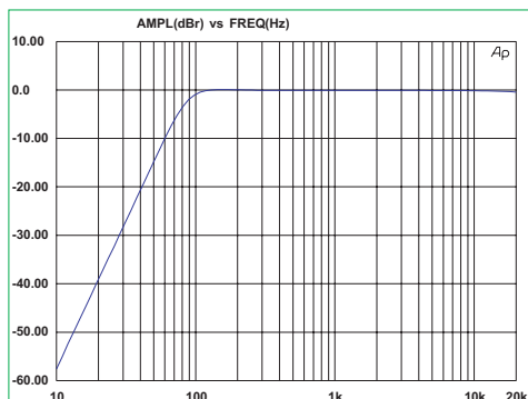
100 Гц НЧ-фильтр
