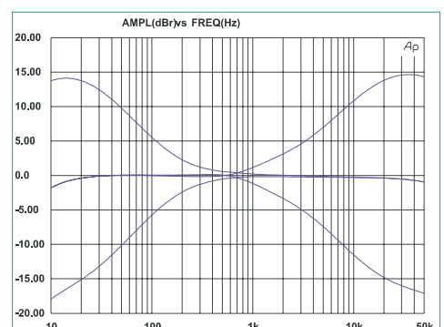
НЧ и ВЧ эквалайзеры
