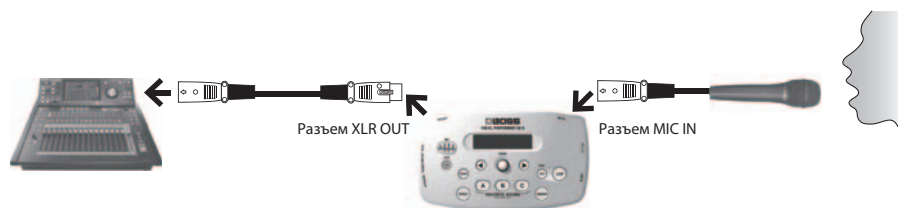
Подключение микрофона через VE-5
